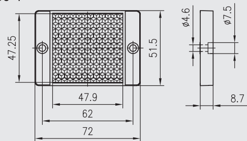
RB50x50-1
