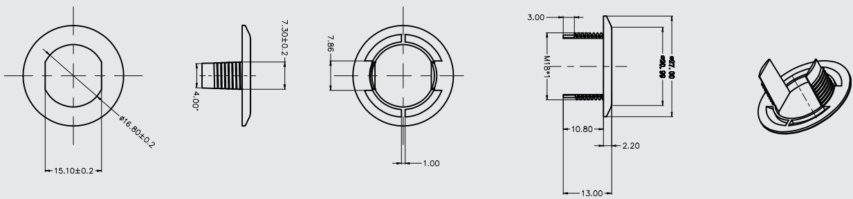
EOG18-1
